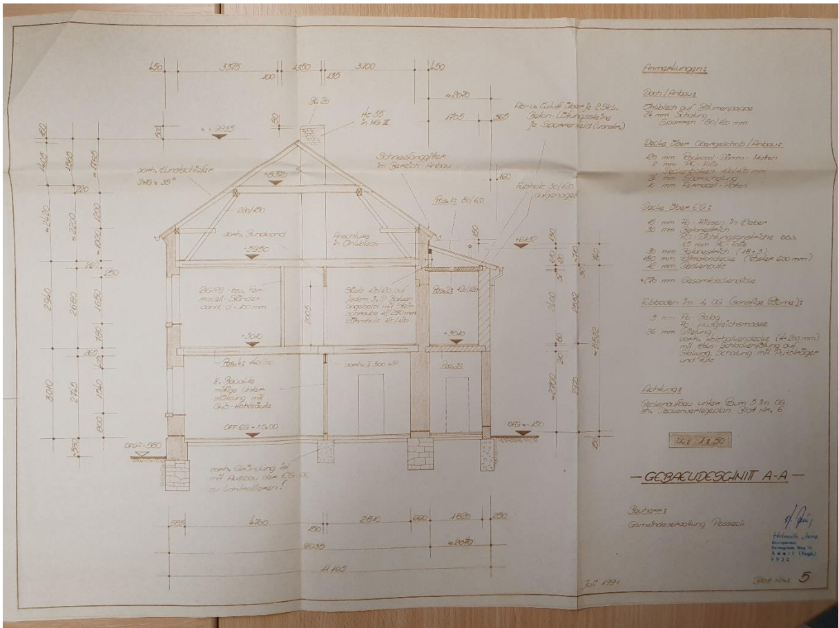
Gebäudeschnitt
